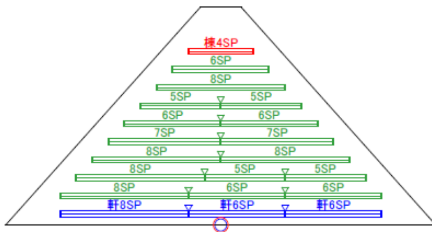
図 1 ステップバー配置参考図
